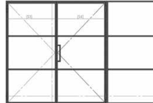
Variante 5: 2-flg. / inkl. Standflügel / inkl. Seitenteil und Zarge
