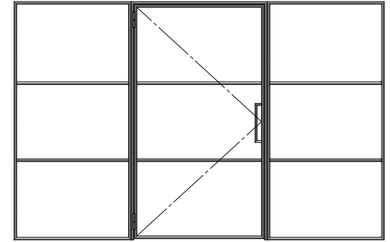
Variante 3: 1-flg. / inkl. Seitenteil links u. rechts
