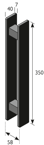
Griffstange Eckig
