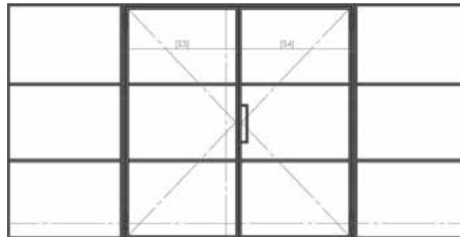
Variante 6: 2-flg. | inkl. Standflügel / inkl. 2 x Seitenteil und Zarge
