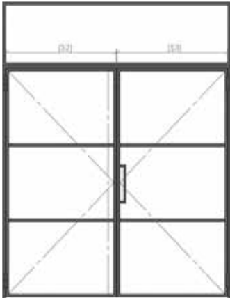
Variante 10: 2-flg. / inkl. Standflügel / inkl. Oberlicht und Zarge
