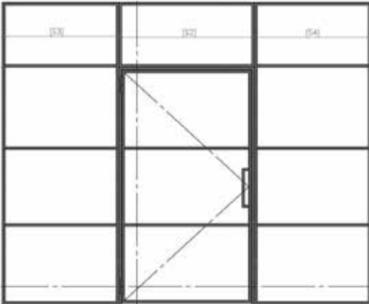
Variante 9: 1-flg. / inkl. Oberlicht / inkl. 2 x Seitenteil und Zarge
