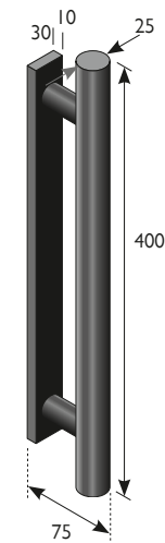
Griffstange Gerundet
