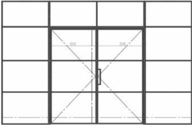
Variante 12: 2-flg. / inkl. Standflügel / inkl. Oberlicht / inkl. 2 x Seitenteil
