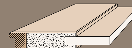
Rahmentür: echte Rahmenbauweise, Füllung eingeschoben
