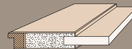
Rahmentür: echte Rahmenbauweise, Füllung eingeschoben
