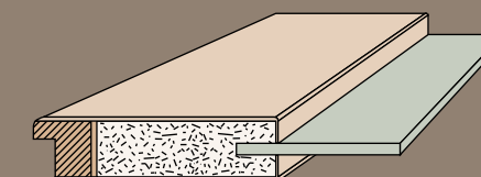
Tür mit Lichtausschnitt: Glas eingeschoben
